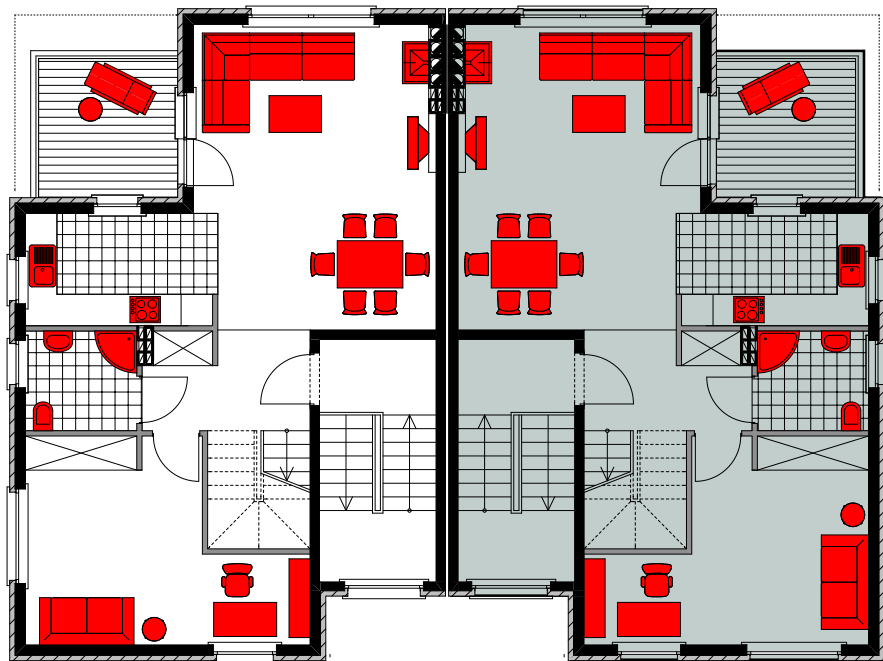
Budynek nr 1, rzut poziomu 1
