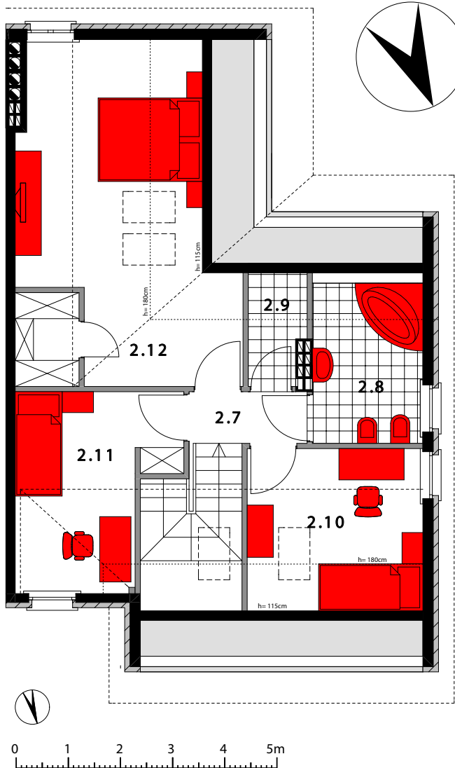
Rzut poziomu II
